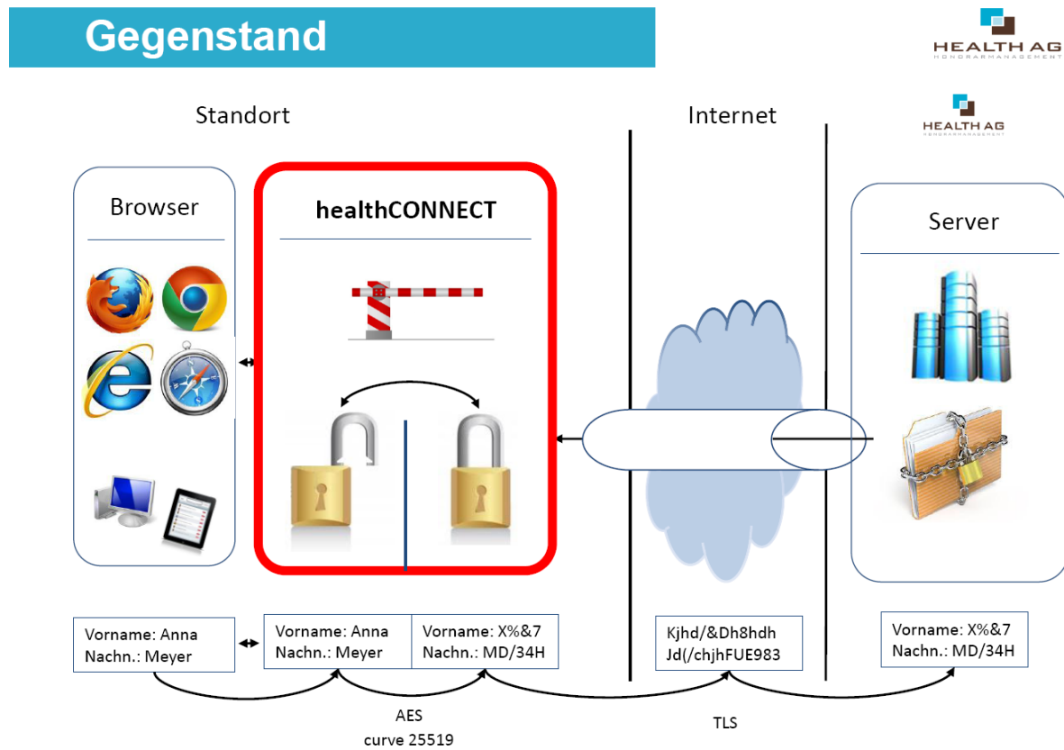
Abbildung 2: Datenfluss und Verschlüsselung von healthCONNECT
